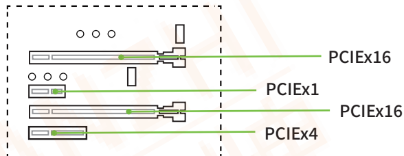
图2-4 PCI扩展插槽
