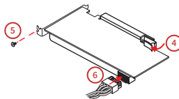
图2-11 显卡安装
