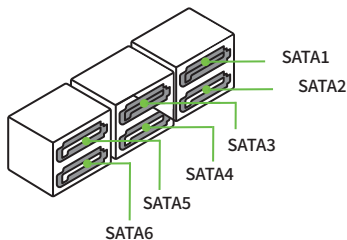
图2 -12 SATA接口
