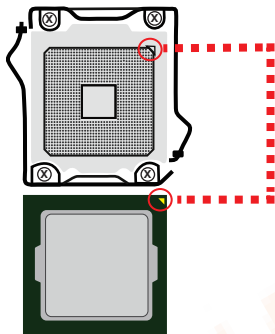
图2-7 CPU底座安装
